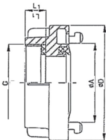
AW 710 Storz Festkupplung Storz adapter
